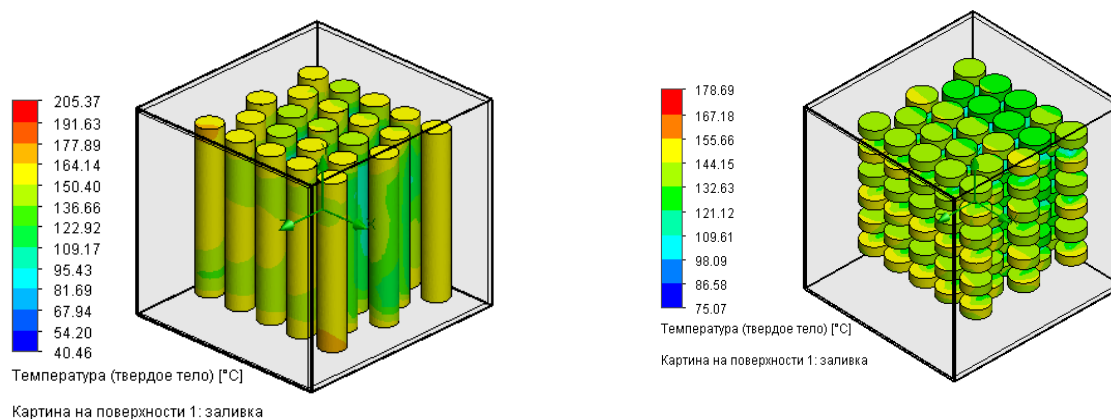
Рисунок 2 – Примеры прогнозного распределения температурного поля поверхности обрабатываемых изделий
