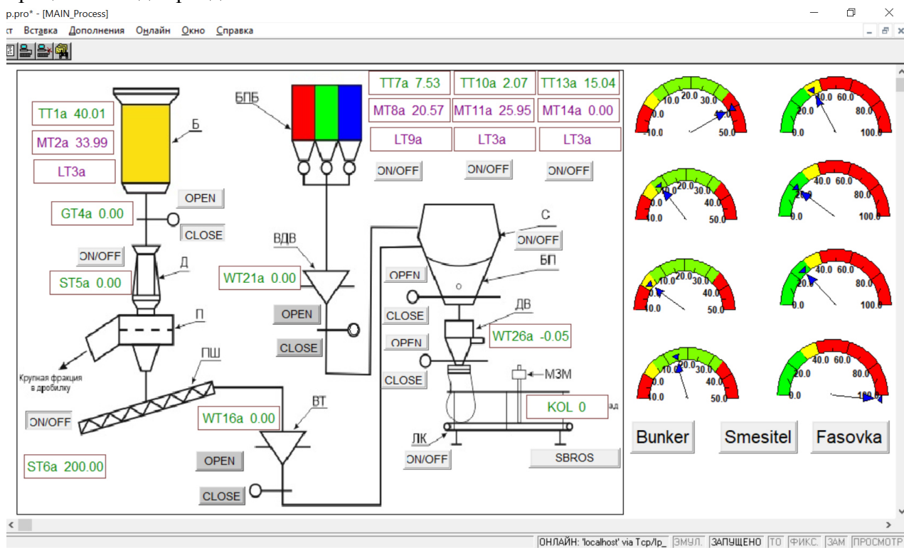
Рисунок 2 – Автоматизированное место оператора (главное окно)
