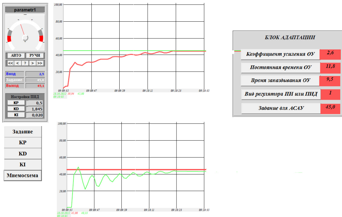
Рисунок 3 – Экран установки параметров регулятора, выбора режима работы
