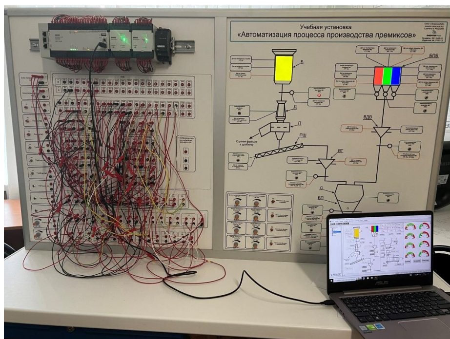
Рисунок 1 – Учебный стенд «Автоматизация процесса производства премиксов»
