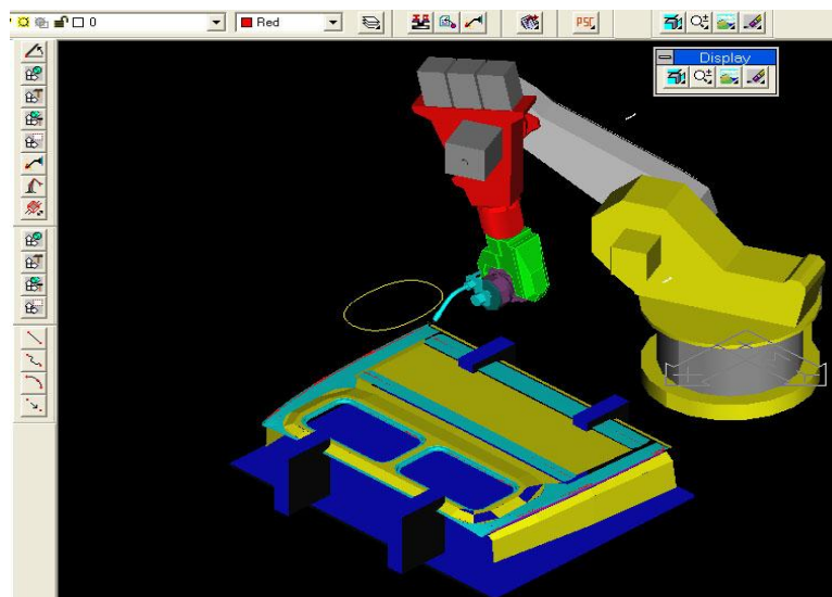
Рисунок 3 – Моделирования движения робота манипулятора в среде виртуального моделирования объектов автоматизации и мехатронных устройств
