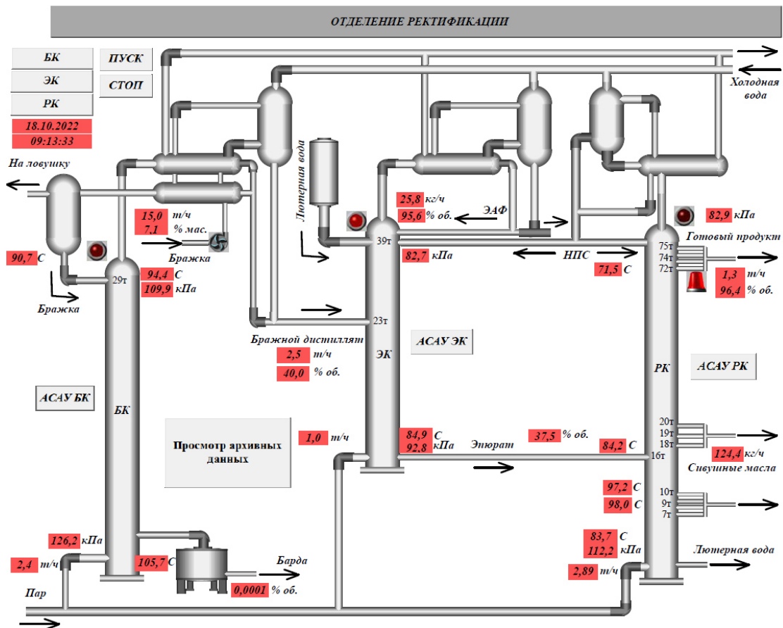
Рисунок 2 – Мнемосхема процесса ректификации
